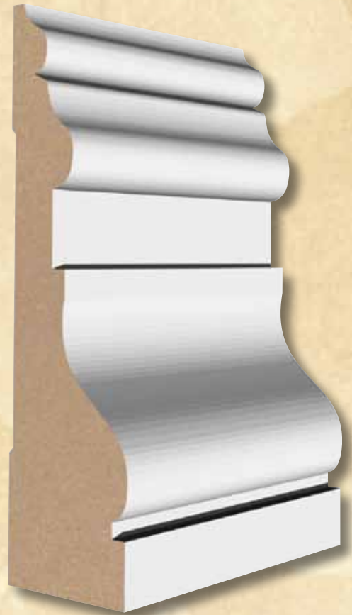
GS425 MDF 1-3/16x4-1/4
